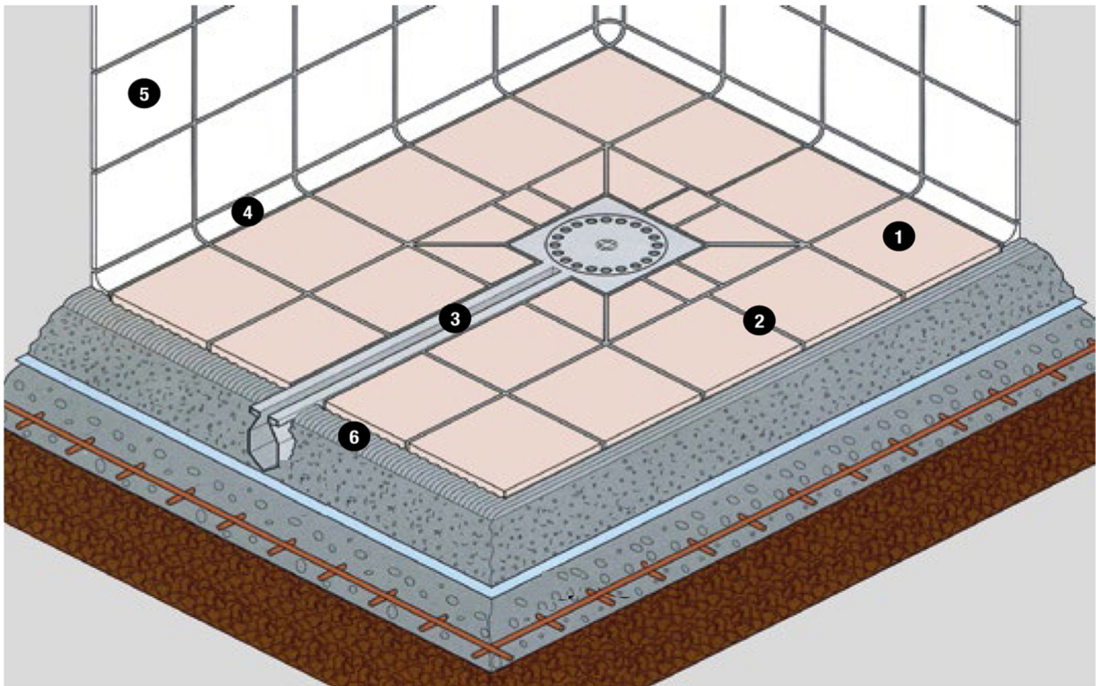
Δείγμα με κούρμπα υγιεινής και ανοξειδωτο κανάλι σχισμής
