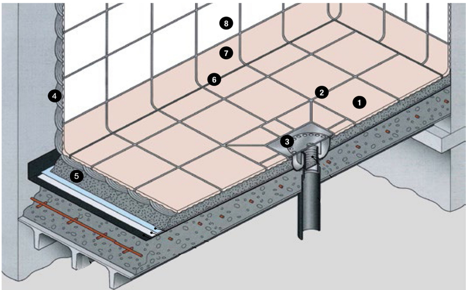
Δείγμα με σοβατεπί κούρμπα υγιεινής και ανοξειδωτο τετράγωνο σιφώνι
